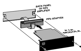
Fig. 8.2 Installing a PIP Module
